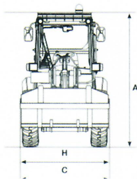
Radlader mit Standardschaufel und Standardbereifung (Frontansicht)
