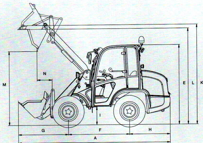
Mit Standardschaufel und Standardbereifung (Seitenansicht)
