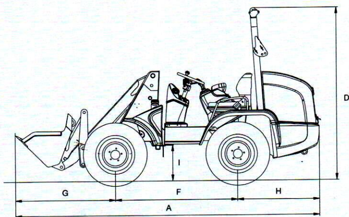
Mit Standardschaufel und Standardbereifung (Seitenansicht)
