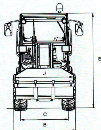
Mit Standardschaufel und Standardbereifung (Frontansicht)
