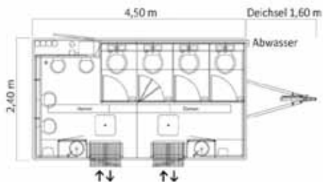
Technische Zeichnung
