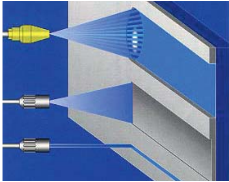
rotierende Punktstrahldüse
