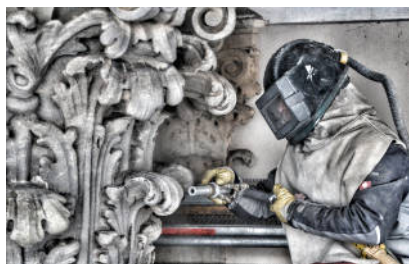
Trockenstrahlen mit MEOS S2 + NDW - Deutsche Staatsoper -
