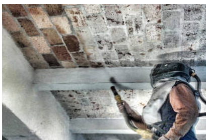
Trockenstrahlen mit MEOS S2
