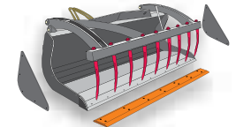
MEHRZWECKSCHAUFEL MIT NIEDERHALTER
