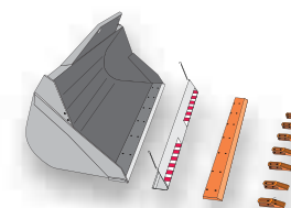
ERDSCHAUFEL MIT SCHNEIDKANTE UND ZÄHNEN
